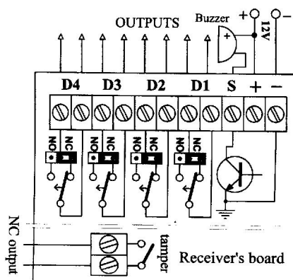
Схема подключения.
