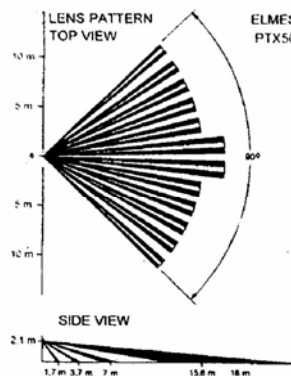
Рис. 2 Диаграмма направленности.
